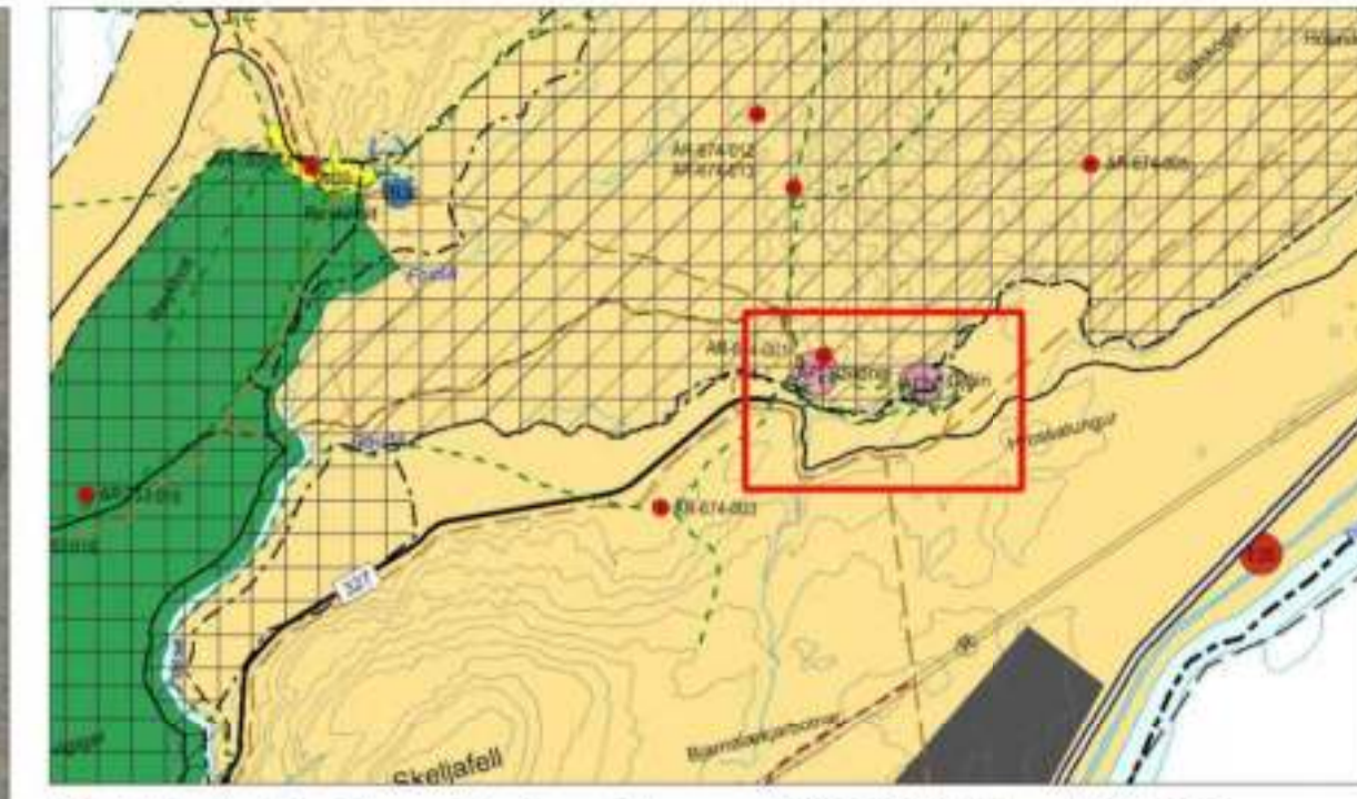
Aðalskipulag Skeiða- og Gnúpverjahrepps 2017-2029. Mkv. 1:50.000.
